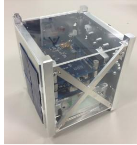
OPUSAT-KIT
