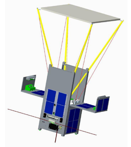
OPUSAT-II
