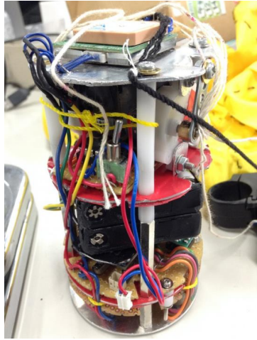
Tsukushi
